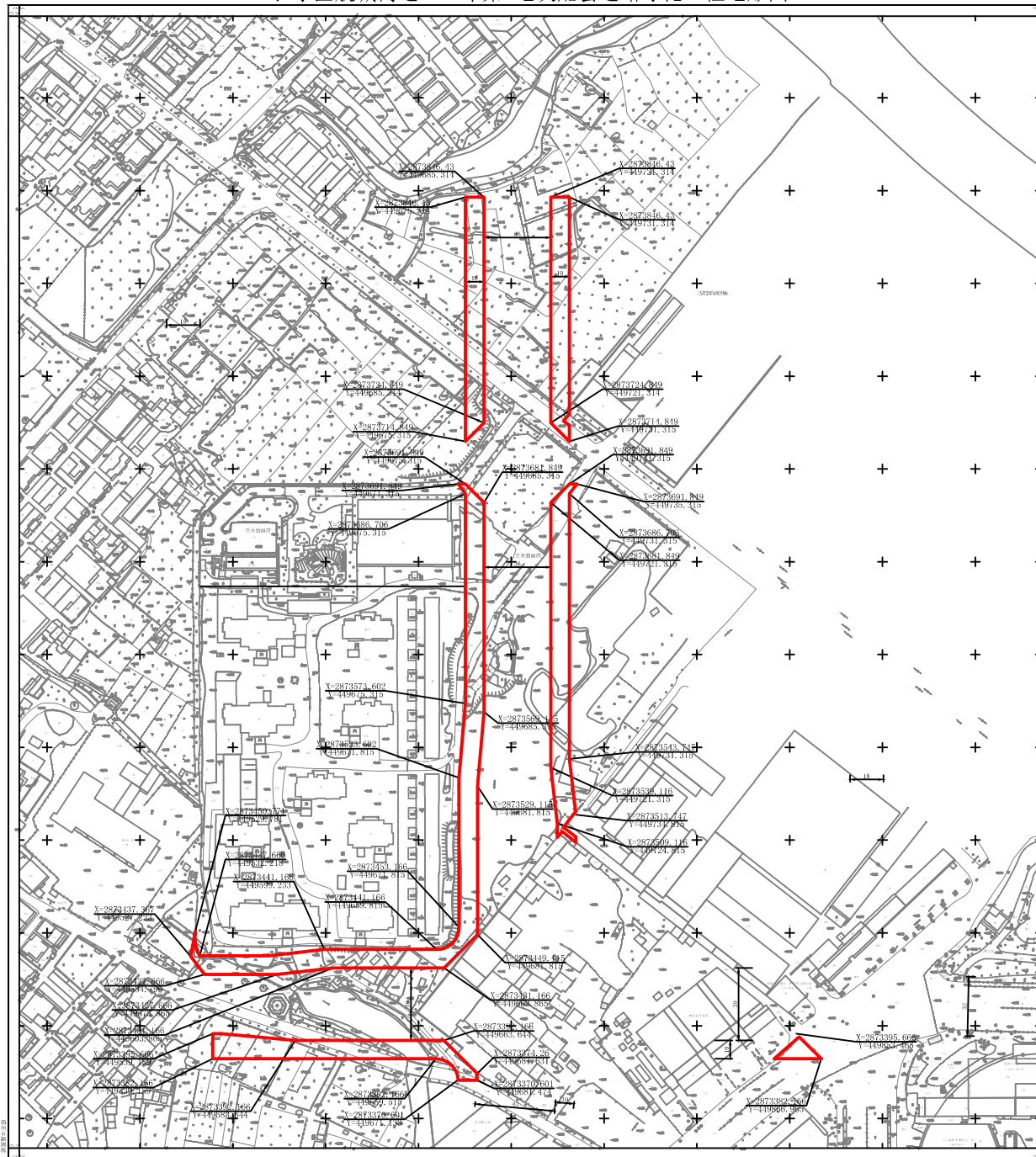
长乐区航城街道2019年第5地块配套道路绿化工程地形图
